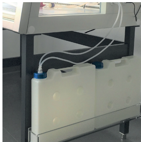
Halterung Sicherheitswerkbank für 2 x 5 l Tanks für die Innenseite oder Außenseite am Untergestell schnell und sicher eingehängt
