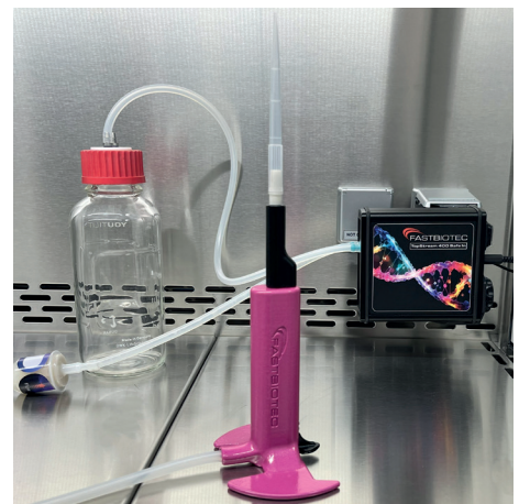
Absaugung direkt in der Sicherheits- werkbank Aspiration directly in the safety cabinet
